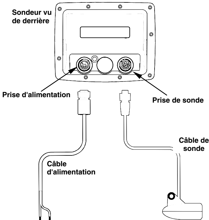
Branchement de sondeur.
