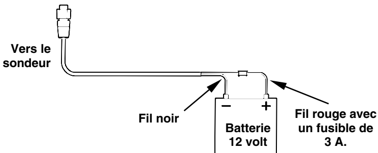
Branchement électrique du sondeur.
