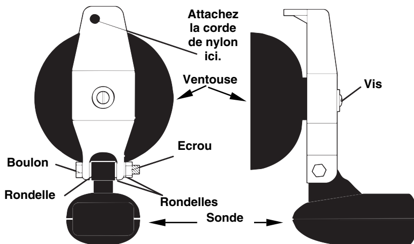
Assemblage de la sonde portatif: Perspective arrière (à gauche) et vue de côté (à droite)
