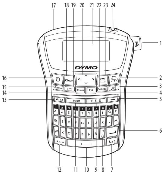
Figure 1 Étiqueteuse électronique LabelManager 220P
