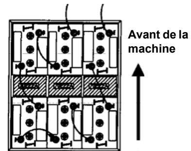
250 Ah, 6 Volts (Batterie n°881317 à liquide) (Batterie n°881318 sèche) Trois (3) entretoises 70222A
