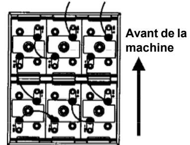
330 Ah, 6 Volts (Batterie n°891384 à liquide) (Batterie n°891385 sèche)
