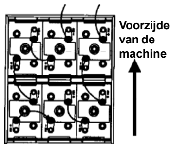
370 AH, 6 Volt (accunr. 40704A Nat) (accunr. 40602A Droog)
