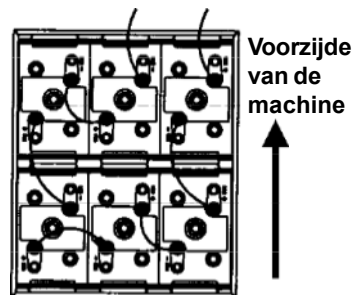
330 AH, 6 Volt (accunr. 891384 Nat) (accunr. 891385 Droog)
