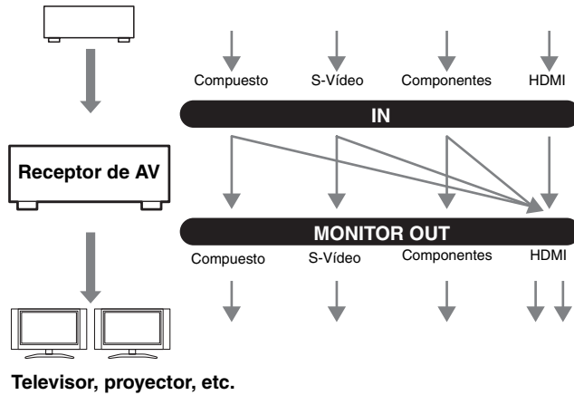
Reproductor de DVD/BD, etc. Gráfico de flujo de señales de vídeo
