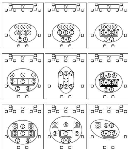
○ : área de audición ①—⑧ : posición de medición
