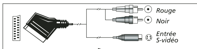
Figure 4 : adaptateur PÉRITELIS-vidéo pour l'écoute ; sens du signal : PÉRITEL → Cinch
