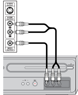
Avant du combiné Graveur DVD + Magnétoscope
