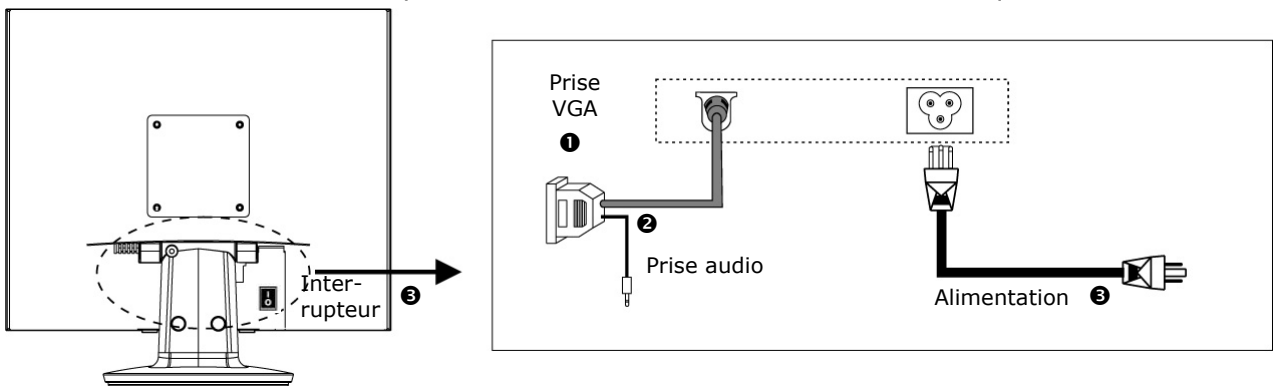
(III.: face arrière de l'écran)
