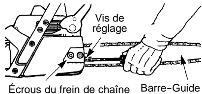
Vis de réglage - 1/4 de tour
