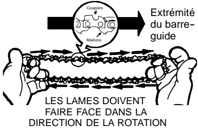
LES LAMES DOIVENT FAIRE FACE DANS LA DIRECTION DE LA ROTATION
