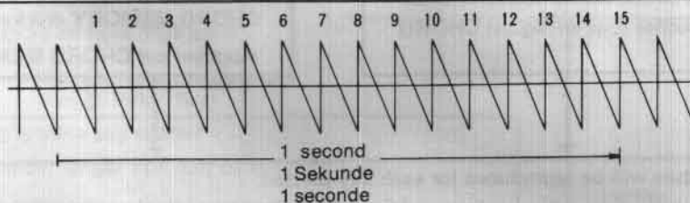
Abb. 1 15Hz-Sägezahnwelle
