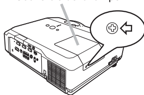
Couvercle de la lampe
