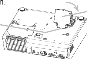
Couvre-filtre pour usage fond vers le haut (avec un filtre à air)
