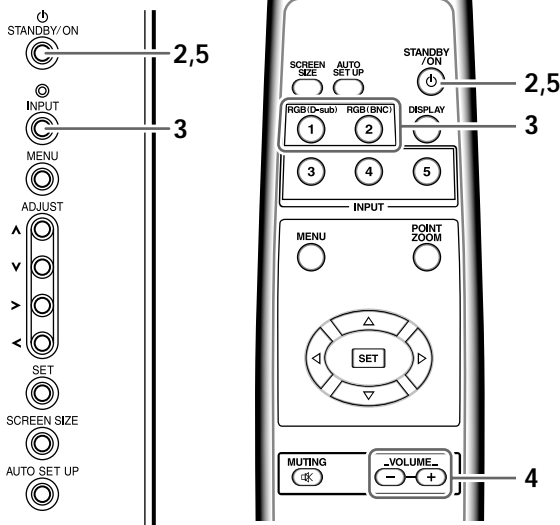
Panneau de commande de l'écran à plasma
