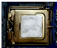
Fig. 1 Veuillez appliquer une couche homogène de pâte de refroidissement sur la surface du processeur installé.
