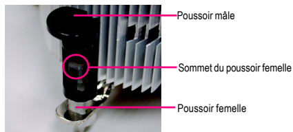
Fig. 2 (en faisant tourner le poussoir dans le sens de la flèche pour retirer le dispositif de refroidissement du processeur, dans le sens contraire pour l'installer) Veuillez vérifier que le sens de la flèche sur le poussoir mâle n'est pas tourné vers l'intérieur avant l'installation. (ces instructions ne sont destinées qu'au ventilateur Intel)
