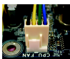
Fig. 6 Pour finir, veuillez fixer le connecteur d'alimentation du dispositif de refroidissement du processeur au ventilateur du processeur situé sur la carte mère.
