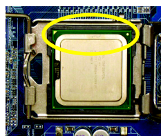
Fig. 3 Notez le petit triangle doré situé au bord du support processeur. Alignez le coin indenté du processeur sur le triangle et insérez délicatement ce dernier dans sa position. (en saisissant fermement le processeur entre le pouce et l'index, placez-la doucement dans le support d'un mouvement rectiligne et vers le bas. Évitez des mouvements de torsion ou de pliage qui pourraient votre matériel au cours de l'installation.)
