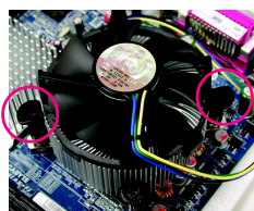
Fig. 3 Placez le dispositif du processeur et assurez-vous que les poussoirs visent l'orifice à poussoir sur la carte mère. Appuyez vers le bas pour pousser les poussoirs diagonalement.
