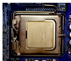
Fig. 4 Une fois que le processeur est correctement inséré, veuillez replacer la plaque de chargement et repousser le levier métallique à sa position d'origine.
