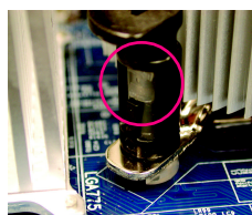
Fig. 4 Veuillez vous assurer que les poussoirs mâle et femelle se rejoignent fermement. (pour des instructions d'installation détaillées, veuillez consulter la section d'installation du dispositif de refroidissement du processeur dans le manuel d'utilisateur)
