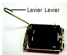
Fig. 1 Soulevez délicatement le levier métallique situé sur le support du processeur en position verticale.
