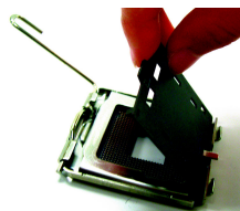
Fig. 2 Retirez le couvercle de plastique sur le support processeur.
