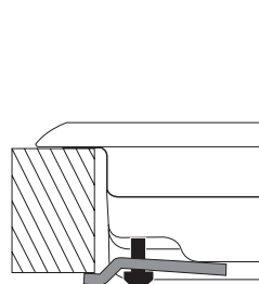
Θέση γάντζου για top H=40mm
