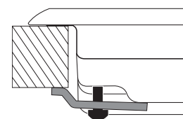
Θέση γάντζου για top H=30mm
