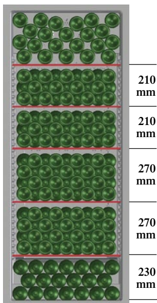
WK 4176 168 bouteilles
