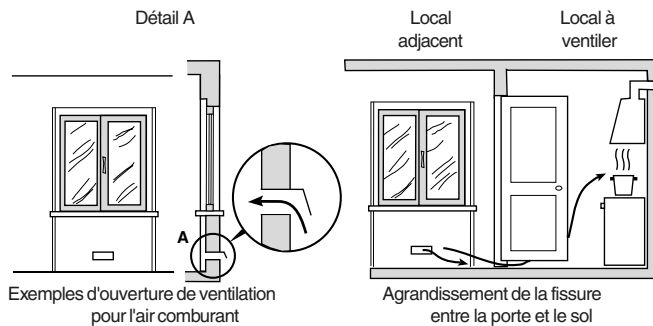
Exemples d'ouverture de ventilation pour l'air comburant
