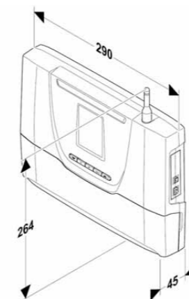
Boîtier de gestion de : • Moduzone Z11 C et Z11 G • Moduzone Z20 C et Z20 G
