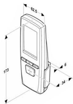
Thermostat d'ambiance • Exacontrol E7R
