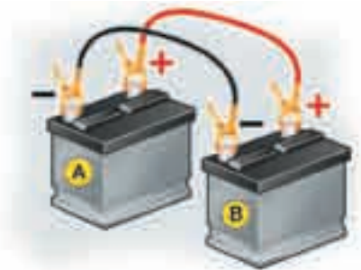
B. Batterie de secours
