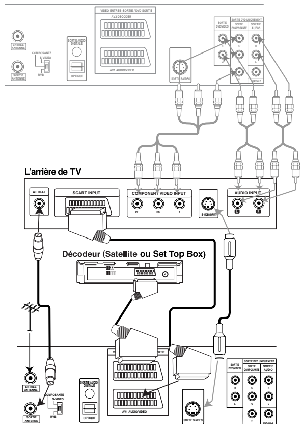
L'arrière de l'appareil (Branchement de base)
