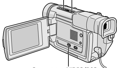
Commutateur VIDEO/DSC (Ouvrir l'écran LCD pour avoir accès à ce commutateur.)
