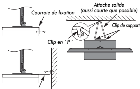
Courroie de fixation
