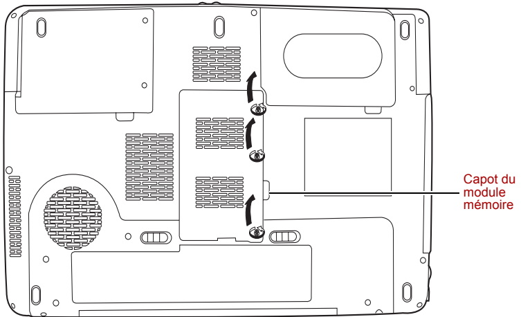
Retrait du couvercle du module mémoire
