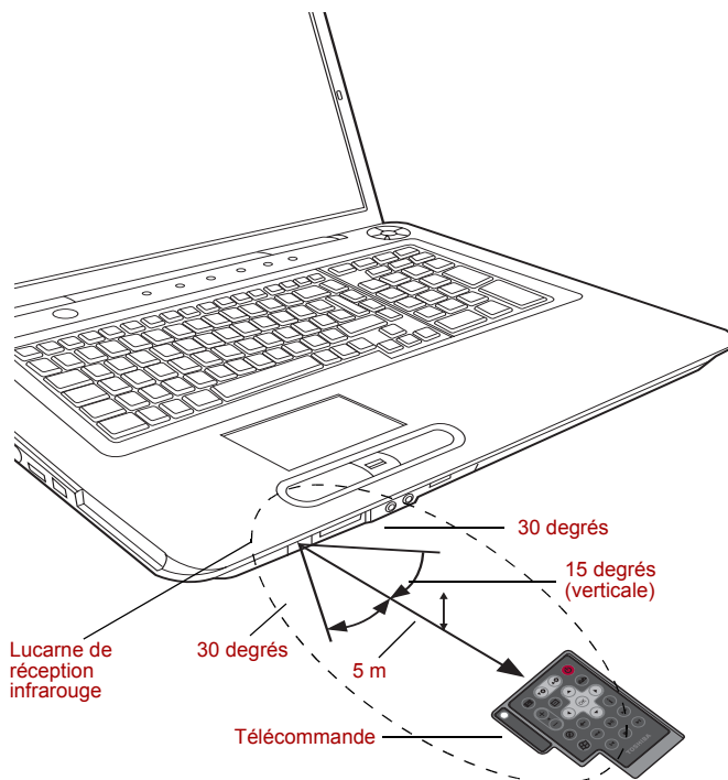
Zone de portée de la télécommande
