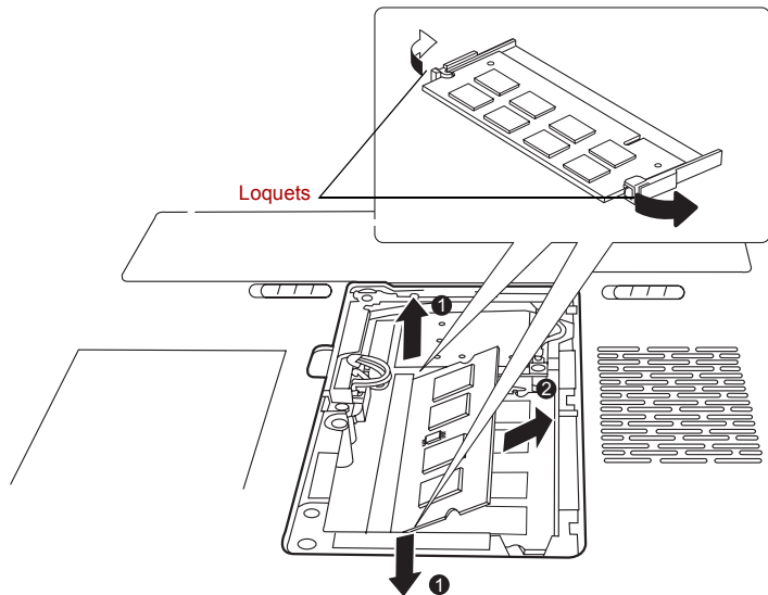
Retrait d'un module mémoire
