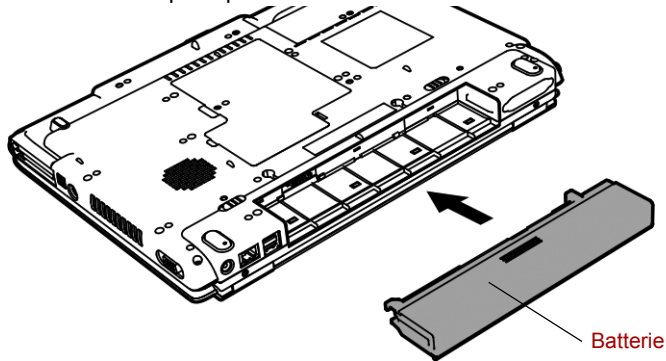
Installation de la batterie principale
