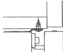
particolare A
