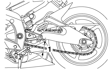
1. Tension de la chaîne de transmission
