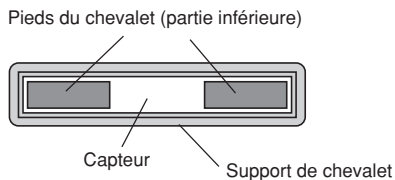
[Positionnement des pieds de chevalet]
