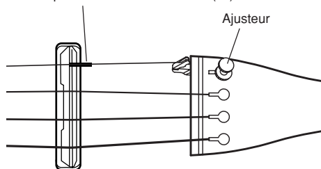
Tube de protection de la 1ère corde (Mi).
