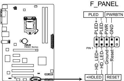
Connecteurs panneau système de la série P8H61
