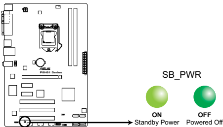
Voyant d'alimentation de la série P8H61
