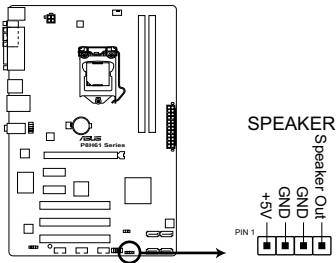
Connecteur pour haut-parleur système de la série P8H61
