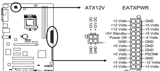
Connecteurs d'alimentation de la série P8H61
