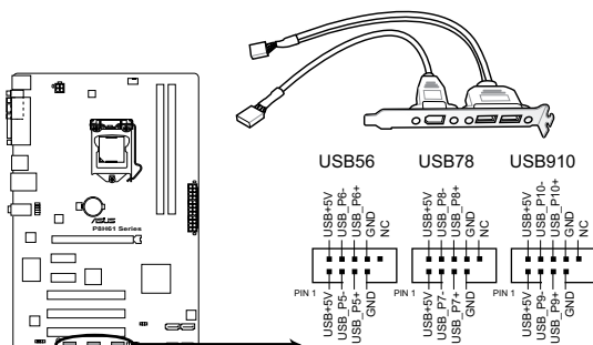
Connecteurs USB de la série P8H61
