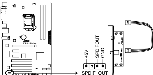
Connecteur audio numérique de la série P8H61
