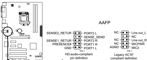
Connecteur pour port audio en façade de la série P8H61
