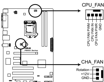
Connecteurs de ventilation de la série P8H61
