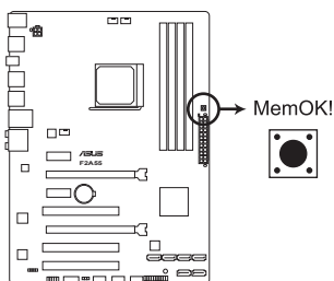
Interrupteur MemOK! de la F2A55
