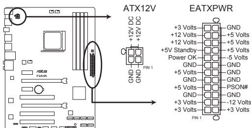
Connecteurs ATX de la F2A55
