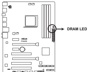
Voyant DRAM de la F2A55
