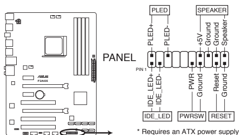
Connecteur système de la F2A55
