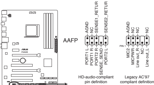
Connecteur pour port audio en façade de la F2A55
