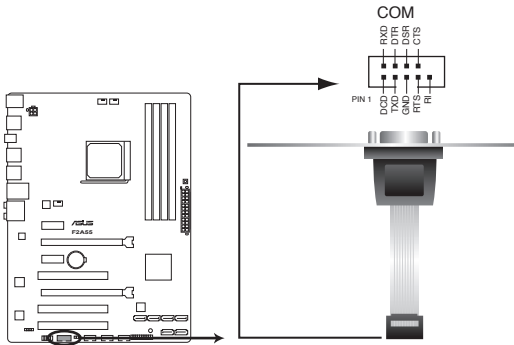
Connecteur pour port COM de la F2A55
