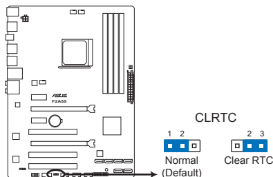
Jumper d'effacement de la mémoire RTC de la F2A55
