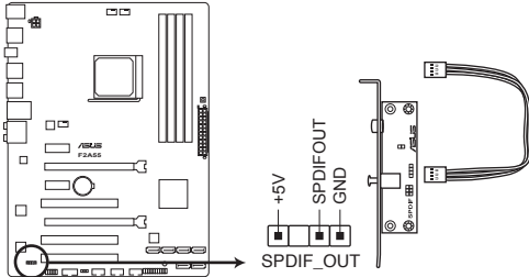
Connecteur audio numérique de la F2A55
