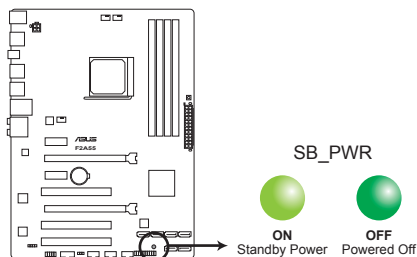
Voyant d'alimentation de la F2A55
