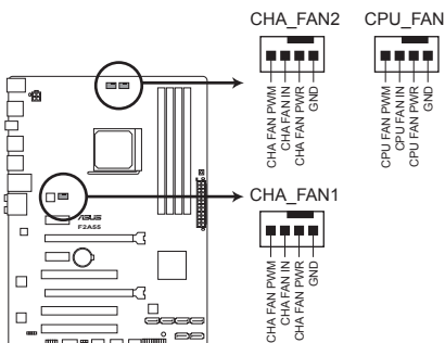
Connecteurs de ventilation de la F2A55
