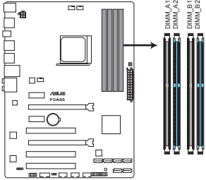
Sockets DIMM DDR3 de la F2A55
