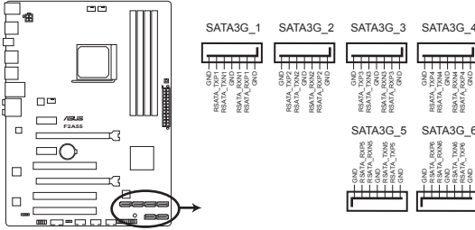
Connecteurs SATA de la F2A55
