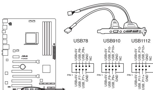
Connecteurs USB 2.0/1.1 de la F2A55
