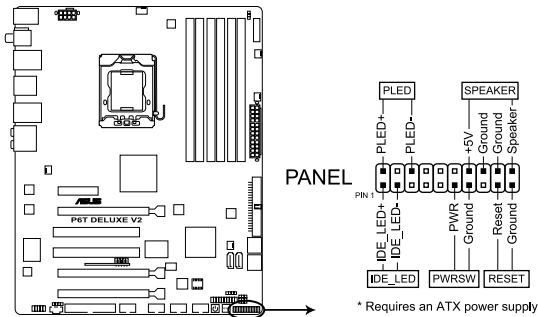
Connecteur système de la P6T Deluxe V2
