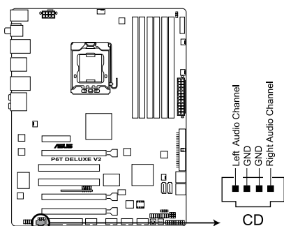
Connecteur audio pour lecteur optique de la P6T Deluxe V2
