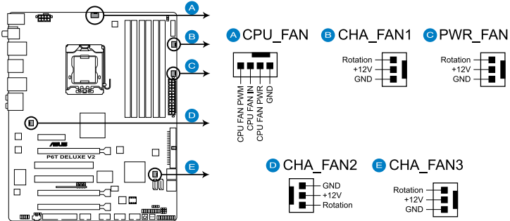
Connecteurs de ventilation de la P6T Deluxe V2
