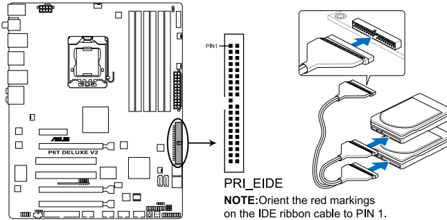
Connecteur IDE de la P6T Deluxe V2
