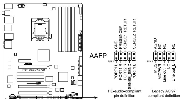
Connecteur audio du panneau avant de la P6T Deluxe V2
