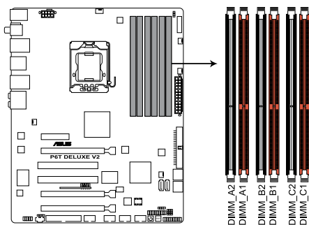
Sockets DIMM DDR3 de la P6T Deluxe V2
