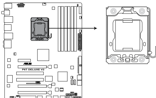
Socket 1366 du CPU de la P6T Deluxe V2
