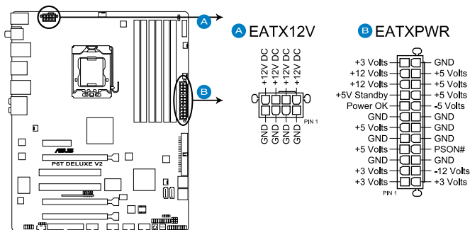
Connecteurs ATX de la P6T Deluxe V2
