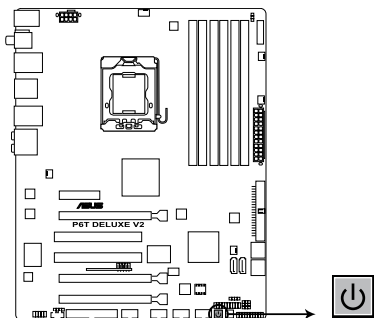
Interrupteur d'alimentation de la P6T Deluxe V2
