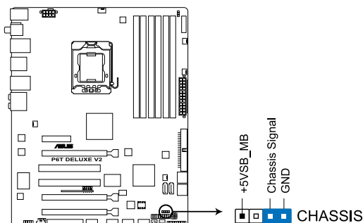
Connecteur d'intrusion châssis de la P6T Deluxe V2
