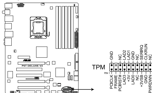
Connecteur TPM de la P6T Deluxe V2
