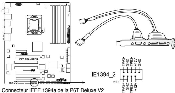
Connecteur IEEE 1394a de la P6T Deluxe V2
