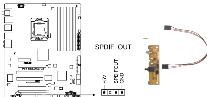
Connecteur audio numérique de la P6T Deluxe V2
