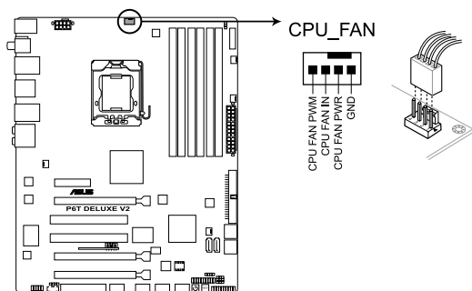
Connecteur CPU_FAN de la P6T Deluxe V2
