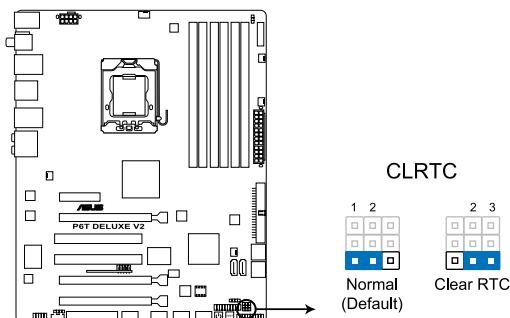
Clear RTC RAM de la P6T Deluxe V2
