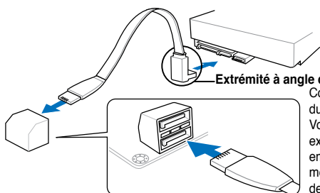
Connecteurs SATA de la P6T Deluxe V2
