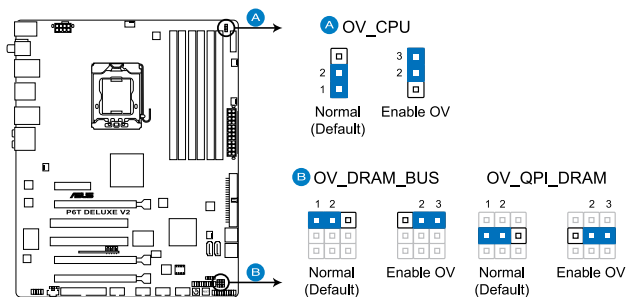
Paramètres de surtension de la P6T Deluxe V2
