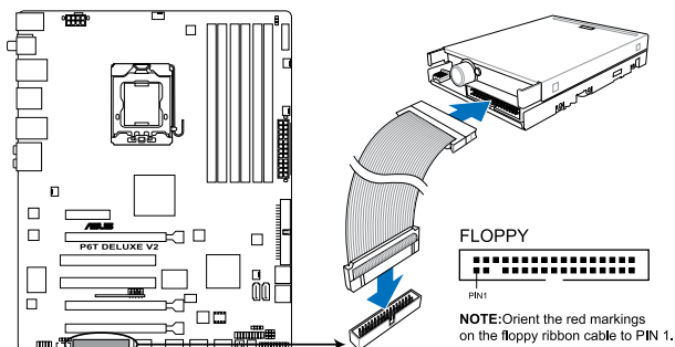
Connecteur pour lecteur de disquettes de la P6T Deluxe V2
