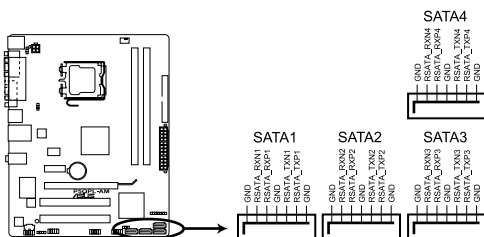
Connecteurs SATA de la P5QPL-AM
