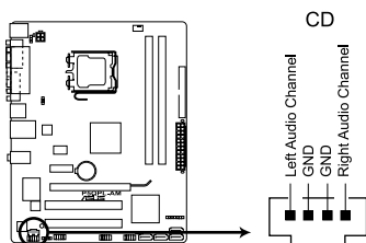
Connecteur audio pour lecteur optique de la P5QPL-AM
