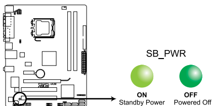
LED embarquée de la P5QPL-AM
