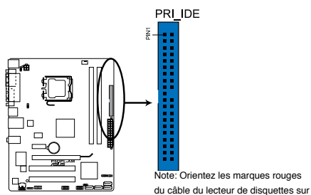
Connecteur IDE de la P5QPL-AM
