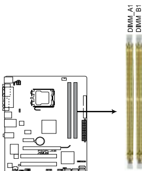
Sockets DIMM DDR2 de la P5QPL-AM
