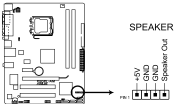
Connecteur haut-parleur d'alerte de la P5QPL-AM
