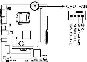
Connecteur CPU_FAN de la P5QPL-AM
