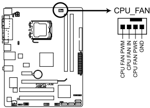
Connecteurs de ventilation de la P5QPL-AM
