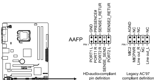
Connecteur audio du panneau avant de la P5QPL-AM
