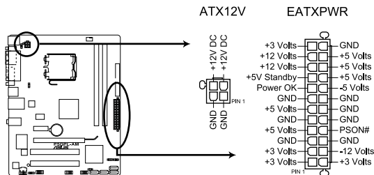
Connecteurs ATX de la P5QPL-AM
