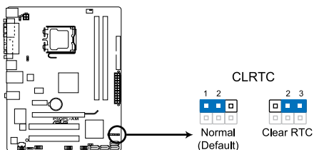
Clear RTC RAM de la P5QPL-AM
