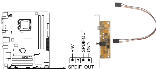
Connecteur audio numérique de la P5QPL-AM
