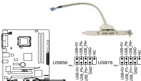
Connecteurs USB 2.0 de la P5QPL-AM
