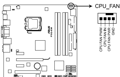
Connecteur CPU_FAN de la P5Q-EM
