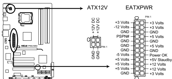
Connecteurs ATX de la P5Q SE2
