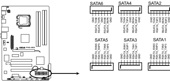
Connecteurs SATA de la P5Q SE2
