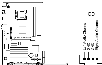
Connecteur audio pour lecteur optique de la P5Q SE2
