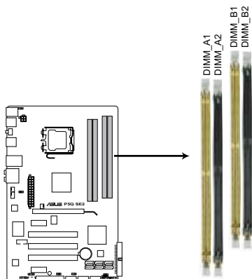
Sockets DIMM DDR2 de la P5Q SE2
