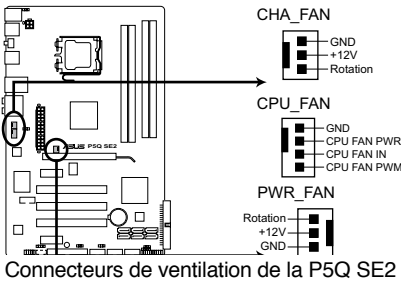
Connecteurs de ventilation de la P5Q SE2
