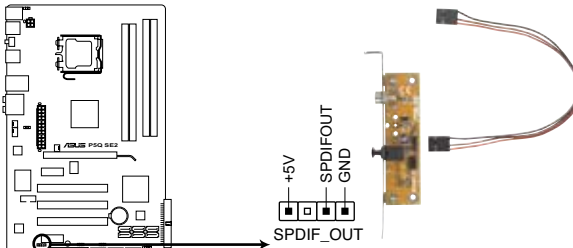
Connecteur audio numérique de la P5Q SE2
