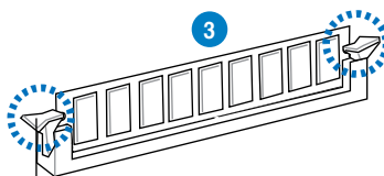
Clip de rétention verrouillé
