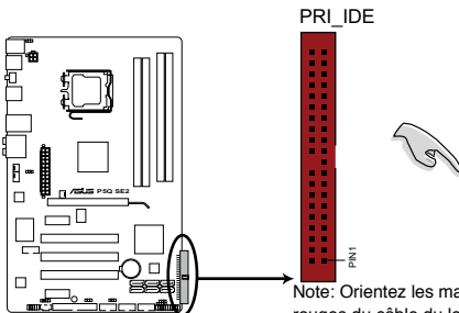
Connecteur IDE de la P5Q SE2
