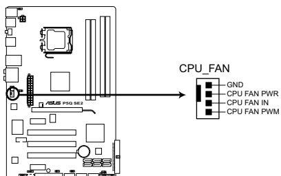
Connecteur CPU_FAN de la P5Q SE2
