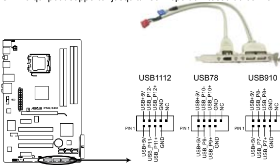
Connecteurs USB 2.0 de la P5Q SE2
