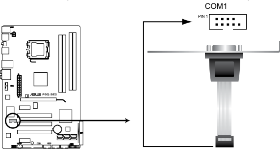
Connecteur port COM de la P5Q SE2
