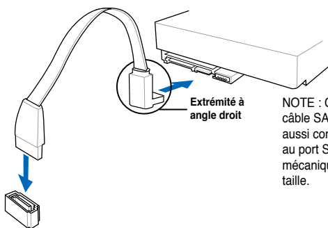
Connecteurs SATA de la P5Q PRO Turbo
