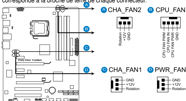
Connecteurs de ventilation de la P5Q PRO Turbo
