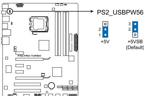
Jumper de sortie de veille via clavier/souris de la P5Q Pro Turbo
