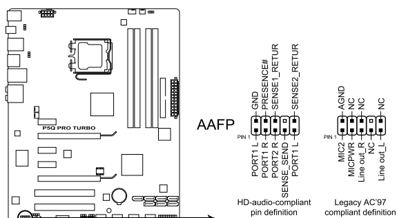
Connecteur audio pour panneau avant de la P5Q PRO Turbo
