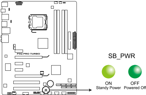
LED embarquée de la P5Q PRO Turbo
