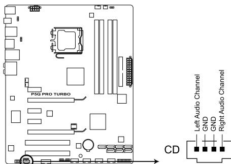
Connecteur audio pour lecteur optique de la P5Q PRO Turbo
