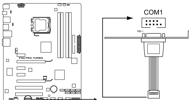
Connecteur port série de la P5Q PRO Turbo
