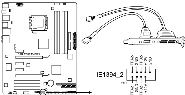
Connecteur port IEEE 1394 de la P5Q PRO Turbo
