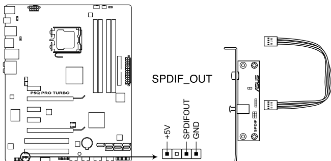
Connecteur audio numérique de la P5Q PRO Turbo
