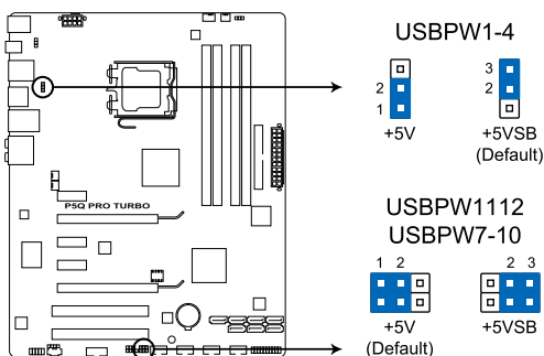
Jumper de sortie de veille via USB de la P5Q Pro Turbo
