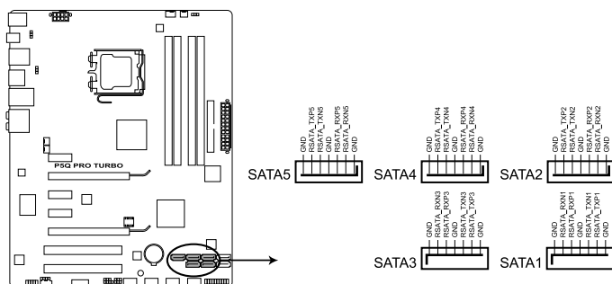
Connecteurs SATA de la P5Q PRO Turbo
