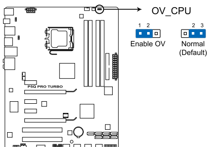
Jumper de surtension de la P5Q PRO Turbo
