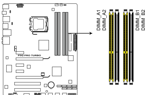
Sockets DIMM DDR2 de la P5Q PRO Turbo
