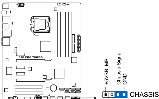
Connecteur d'intrusion châssis de la P5Q PRO Turbo
