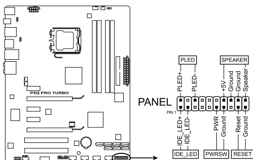
Connecteur panneau système de la P5Q PRO Turbo
