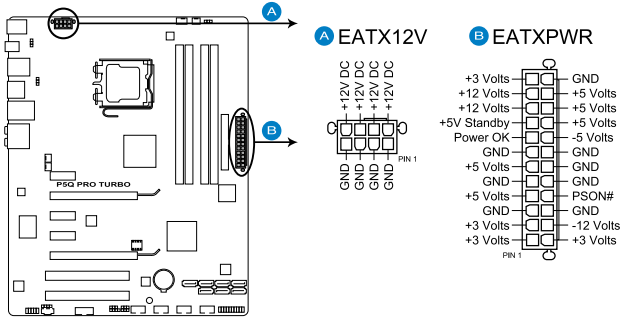
Connecteurs d'alimentation de la P5Q PRO Turbo
