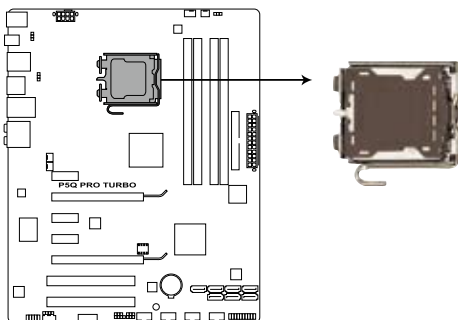
Socket 775 du CPU de la P5Q PRO Turbo
