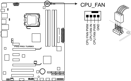
Connecteur CPU_FAN de la P5Q PRO Turbo
