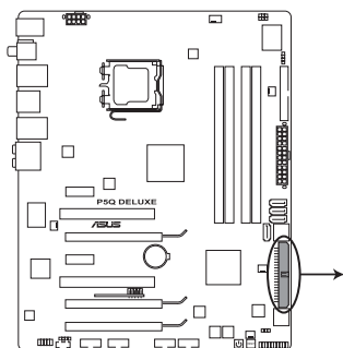
Connecteur IDE de la P5Q Deluxe
