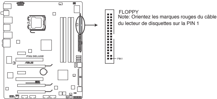
Connecteur pour lecteur de disquettes de la P5Q Deluxe
