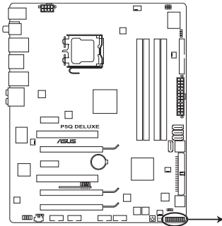
Connecteur panneau système de la P5Q Deluxe
