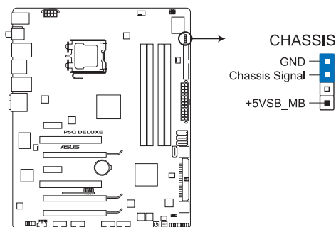
Connecteur du détecteur d'intrusion châssis de la P5Q Deluxe
