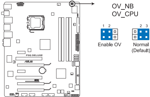
Paramètres de survolage du CPU/Northbridge de la P5Q Deluxe
