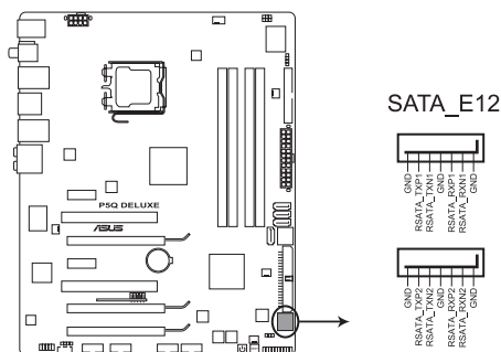
Connecteurs SATA (Silicon Image*) de la P5Q Deluxe
