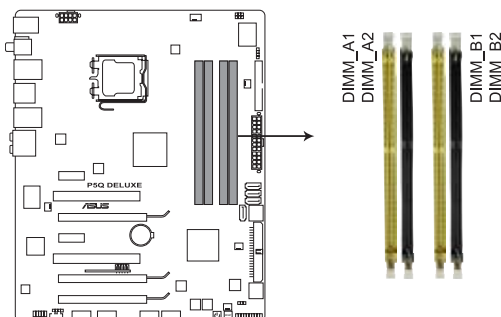
Sockets DIMM DDR2 de la P5Q Deluxe
