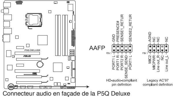
Connecteur audio en façade de la P5Q Deluxe
