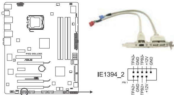
Connecteurs IEEE 1394a de la P5Q Deluxe
