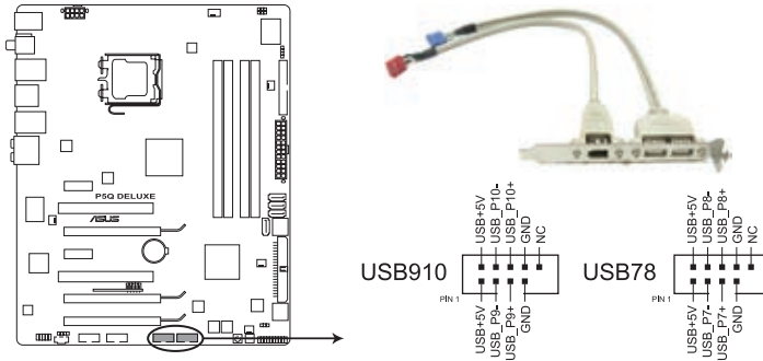
Connecteurs USB 2.0 de la P5Q Deluxe
