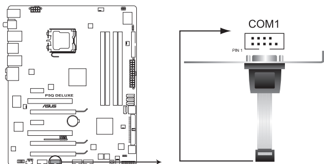
Connecteur du port série (COM1) de la P5Q Deluxe
