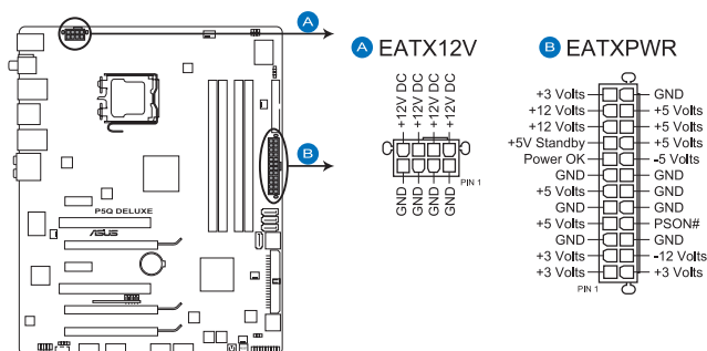
Connecteurs d'alimentation ATX de la P5Q Deluxe
