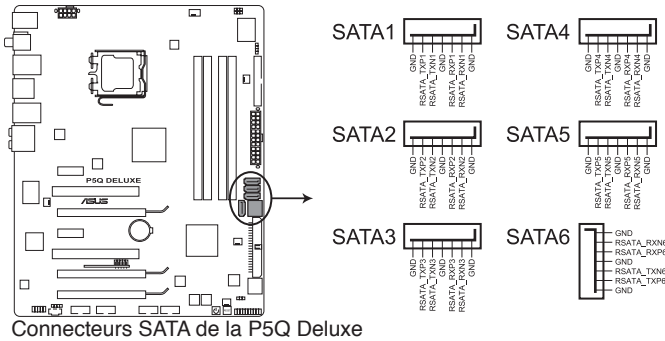
Connecteurs SATA de la P5Q Deluxe
