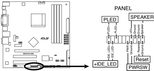
Connecteur système de la M3N78-EM
