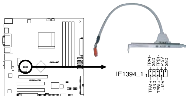
Connecteur IEEE 1394a de la M3N78-EM
