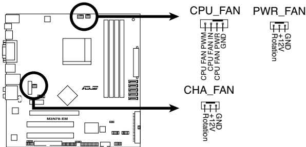
Connecteurs de ventilation de la M3N78-EM
