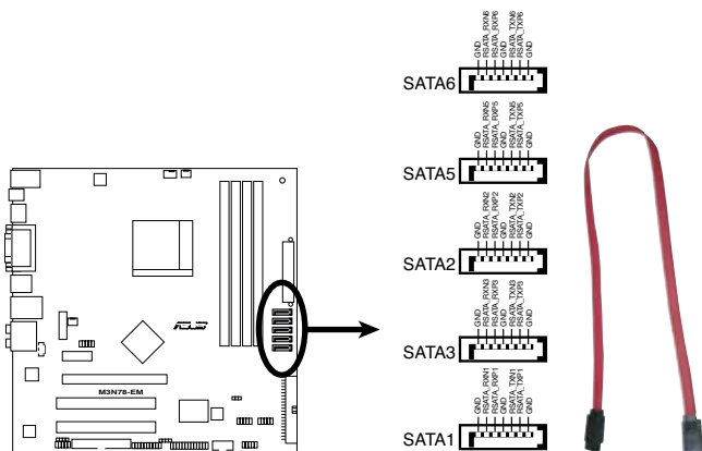
Connecteurs SATA de la M3N78-EM
