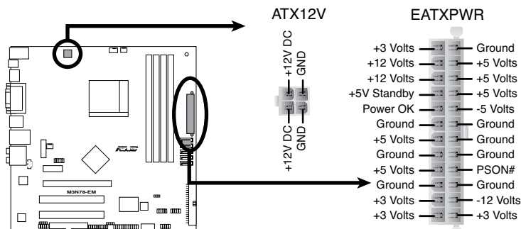
Connecteurs ATX de la M3N78-EM
