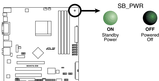
LED embarquée de la M3N78-EM
