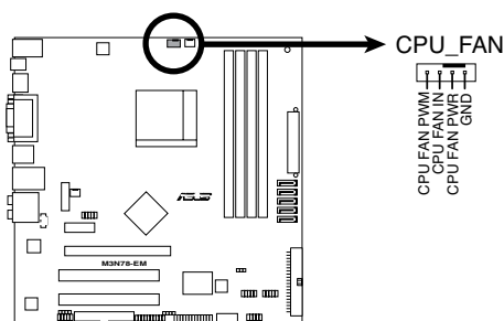
Connecteur du ventilateur du CPU de la M3N78-EM
