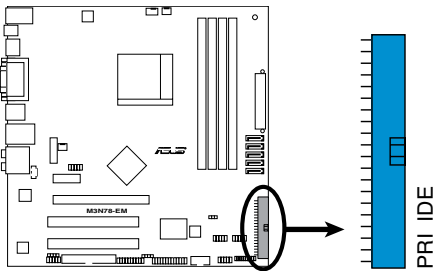
Connecteur IDE de la M3N78-EM
