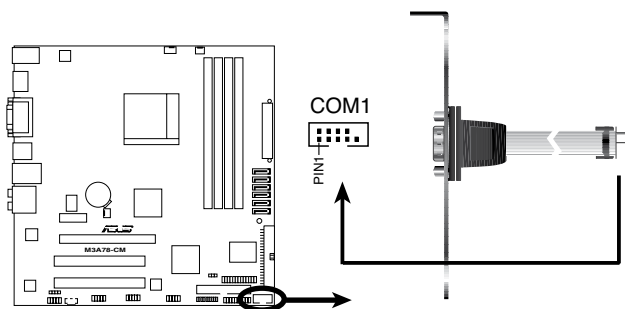
Connecteur port série de la M3A78-CM
