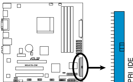
Connecteur IDE de la M3A78-CM
