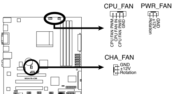
Connecteurs de ventilation de la M3A78-CM
