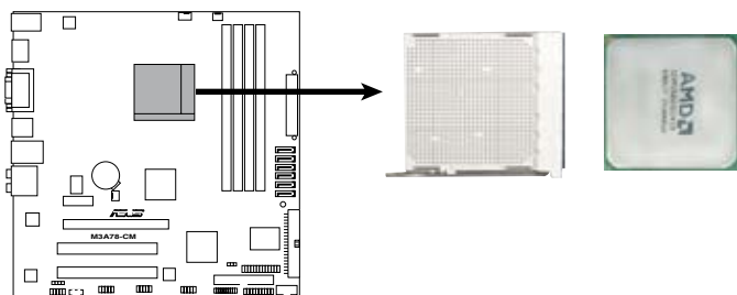
Socket AM2/AM2+ du CPU de la M3A78-CM
