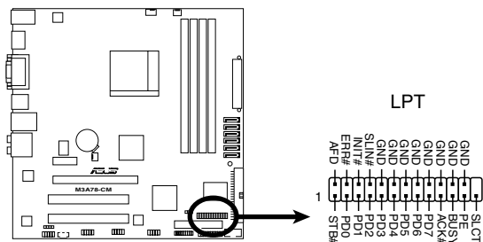
Connecteurs pour port parallèle de la M3A78-CM
