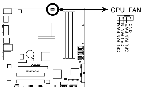
Connecteur du ventilateur du CPU de la M3A78-CM
