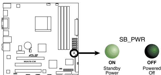
LED embarquée de la M3A78-CM
