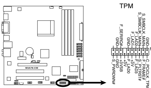
Connecteur TPM de la M3A78-CM
