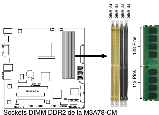
Sockets DIMM DDR2 de la M3A78-CM
