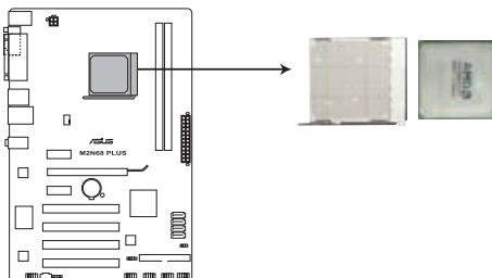
Socket du CPU de la M2N68 PLUS
