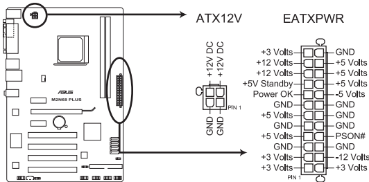
Connecteurs ATX de la M2N68 PLUS
