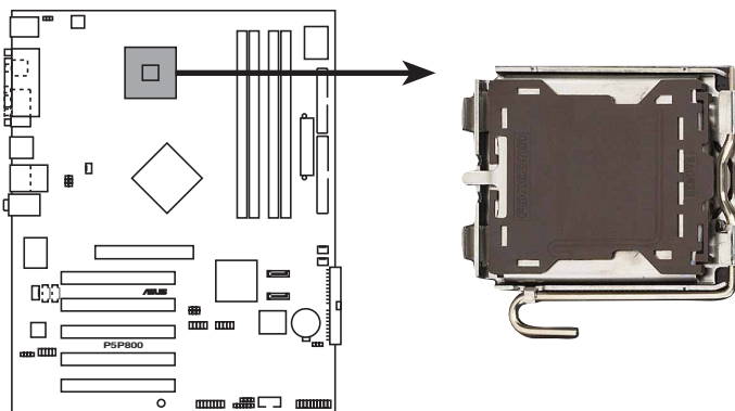
Socket 775 du CPU de la P5P800
