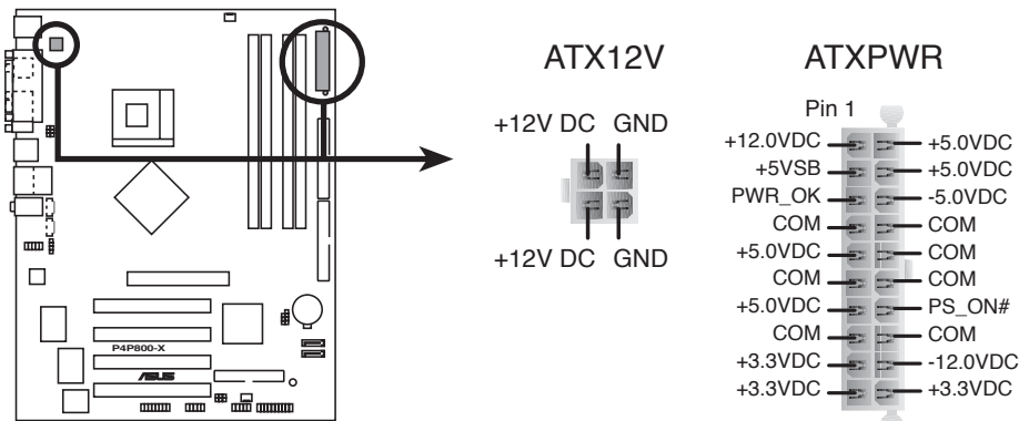
Connecteurs d'alimentation de la P4P800-X
