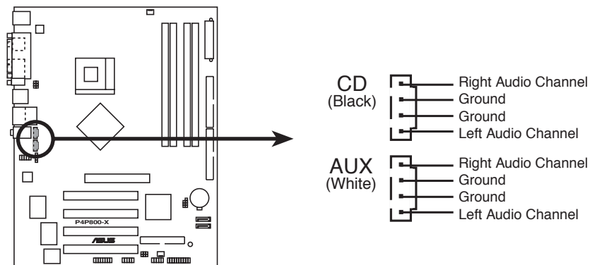
Connecteurs audio internes de la P4P800-X
