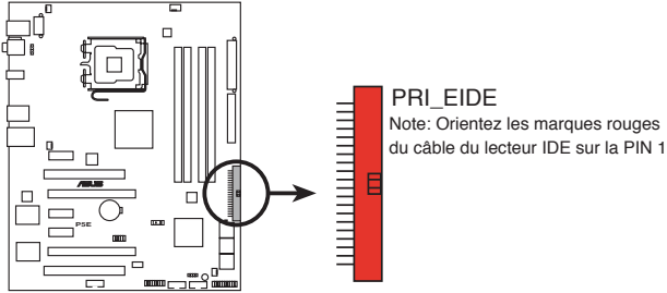
Connecteur IDE de la P5E
