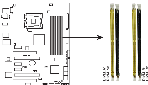
Sockets DIMM DDR2 de la P5E
