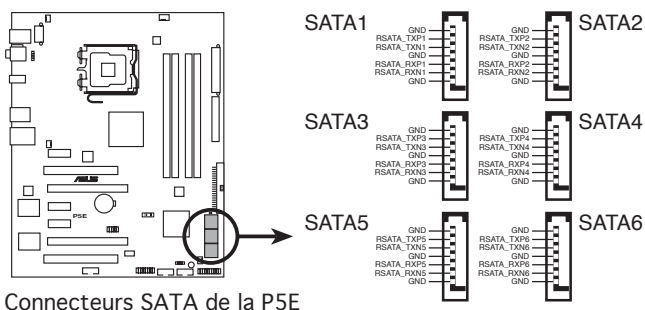
Connecteurs SATA de la P5E
