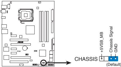
Connecteur chassis intrusion de la P5E
