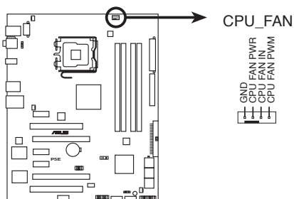
Connecteur CPU_FAN de la P5E
