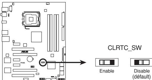
Clear RTC RAM de la P5E
