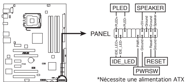
Connecteur système de la P5E
