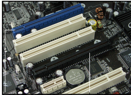
Slot PCI Express Primaire x 16 pour carte graphique unique (bleu)
