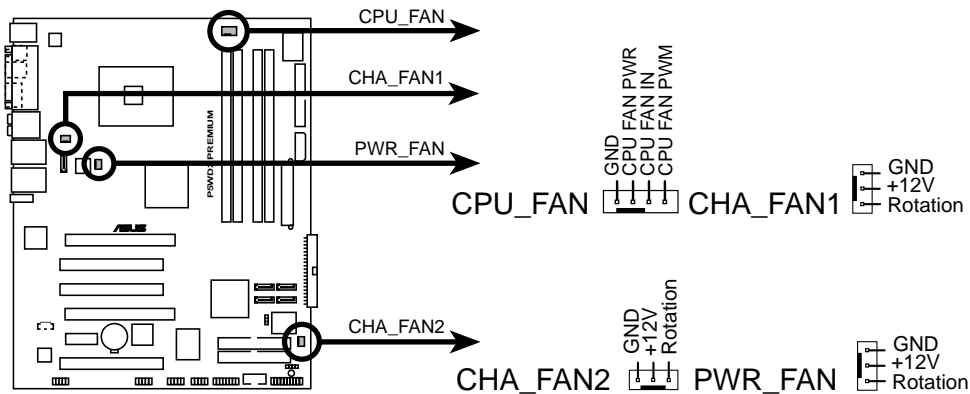
P5WD2 PREMIUM Fan connectors
