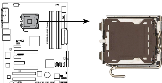
Socket 775 du CPU de la P5N32-SLI SE Deluxe
