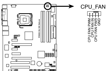
CPU_FAN de la P5N32-SLI SE Deluxe
