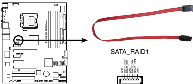
Connecteurs RAID SATA de la P5N32-SLI SE Deluxe
