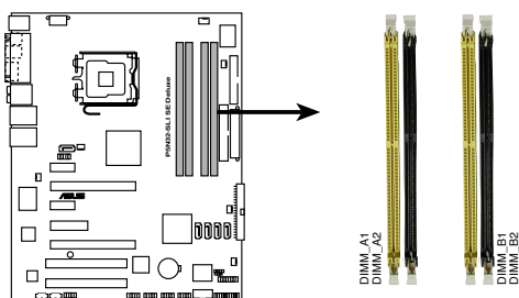
Sockets DIMM DDR2 240 broches de la P5N32-SLI SE Deluxe
