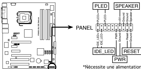
Connecteur System Panel de la P5N32-SLI SE Deluxe
