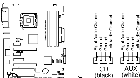
Connecteurs audio internes de la P5N32-SLI SE Deluxe
