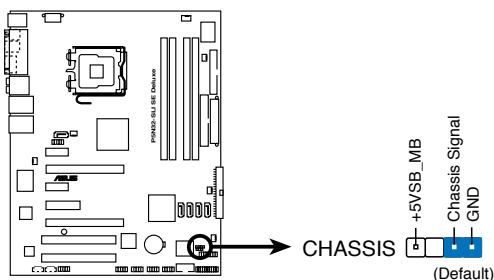
Connecteur Chassis intrusion de la P5N32-SLI SE Deluxe
