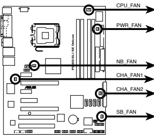
Connecteurs de ventilation de la P5N32-SLI SE Deluxe
