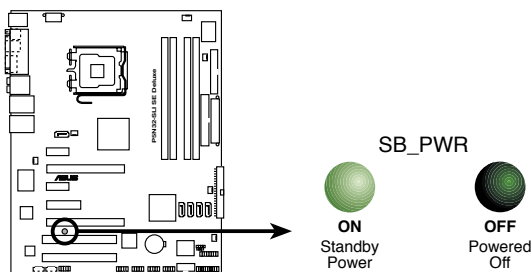
LED embarquée de la P5N32-SLI SE Deluxe
