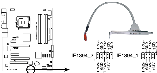
Connecteur IEEE 1394 de la P5N32-SLI SE DELUXE
