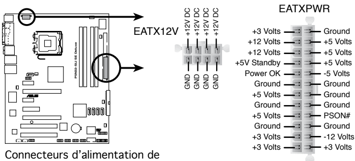
Connecteurs d'alimentation de la P5N32-SLI SE Deluxe
