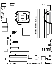
Connecteur pour lecteur de disquettes de la P5N32-SLI SE Deluxe
