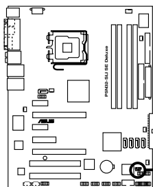
Clear RTC RAM de la P5N32-SLI SE Deluxe
