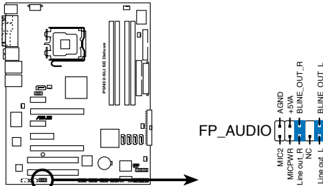
Connecteur Front panel audio de la P5N32-SLI SE DELUXE
