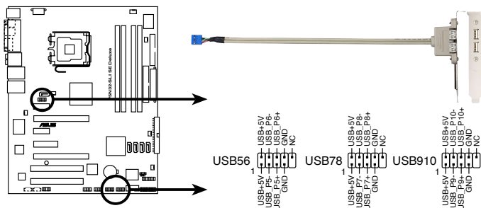
Connecteurs USB 2.0 de la P5N32-SLI SE Deluxe
