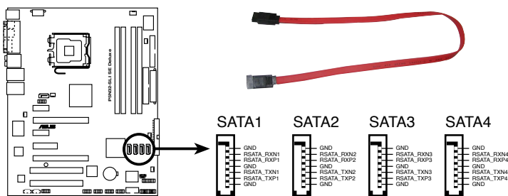
Connecteurs SATA de la P5N32-SLI SE Deluxe
