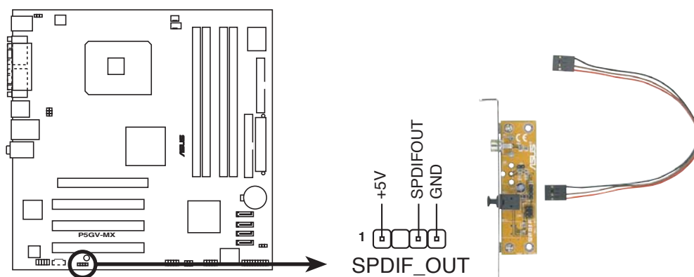
Connecteur audio numérique de la P5GV-MX
