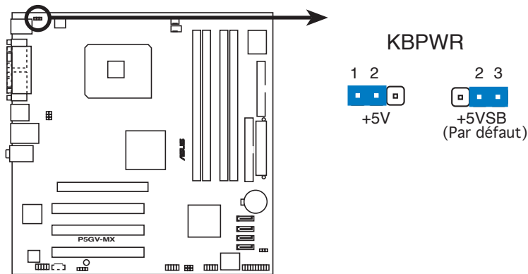
Paramètres d'alimentation du clavier de la P5GV-MX
