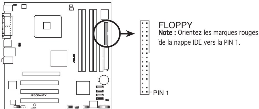
Connecteur lecteur de disquettes de la P5GV-MX
