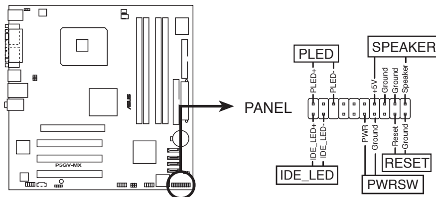
Connecteur System Panel de la P5GV-MX
