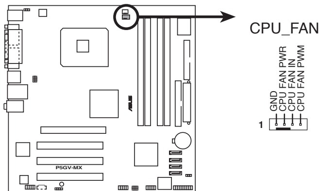
Connecteur CPU_FAN de la P5GV-MX
