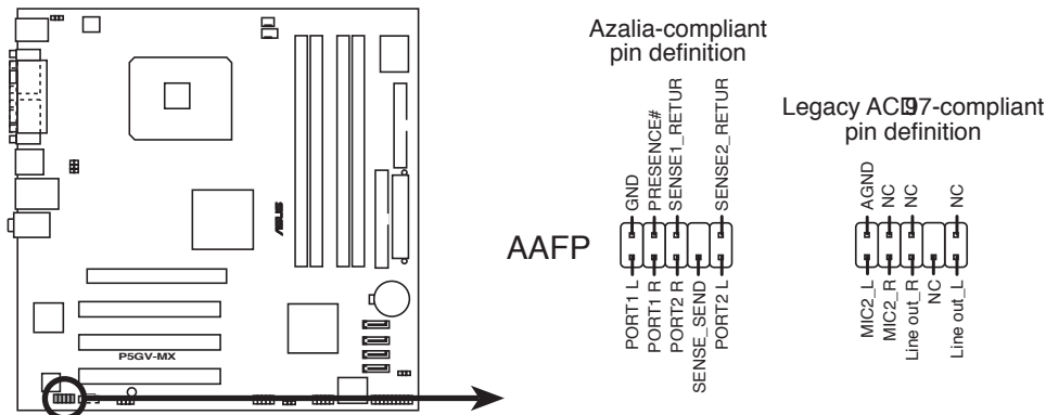
Connecteur Front panel audio de la P5GV-MX
