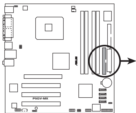
Connecteurs IDE de la P5GV-MX
