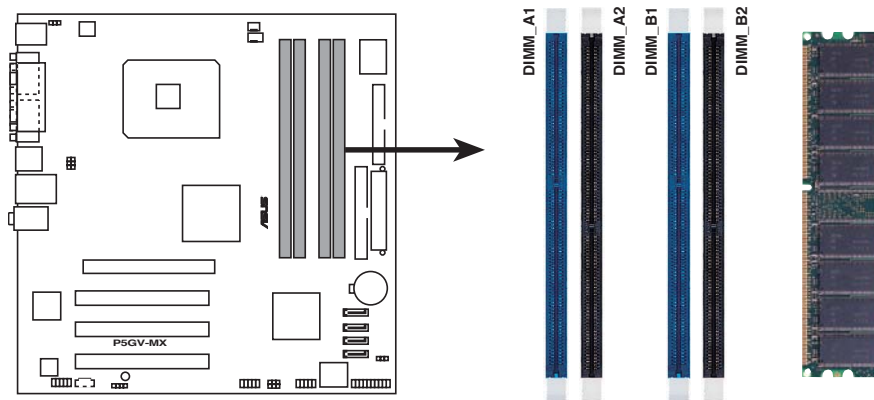
Sockets 184 broches DIMM DDR de la P5GV-MX
