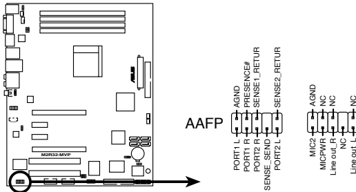
Connecteur Front panel audio de l'M2R32-MVP
