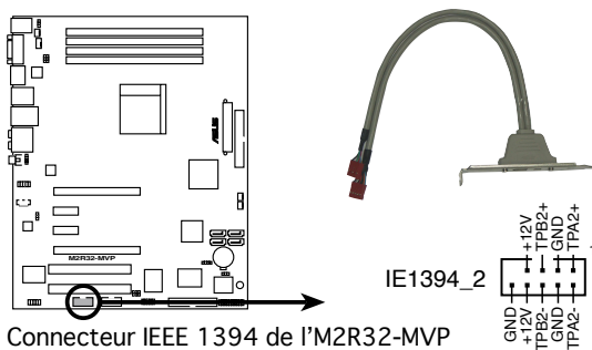
Connecteur IEEE 1394 de l'M2R32-MVP
