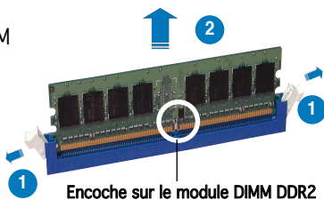
Encoche sur le module DIMM DDR2
