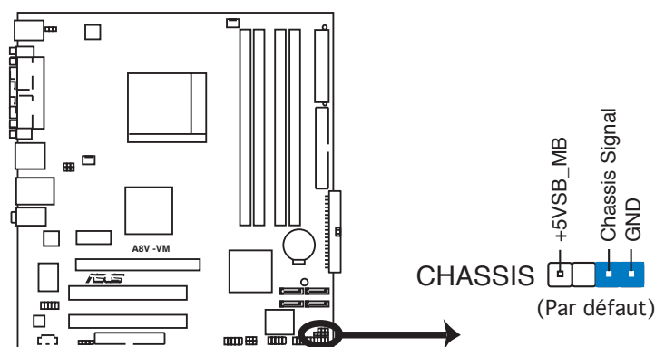
Connecteur Châssis intrusion de l'A8V-VM
