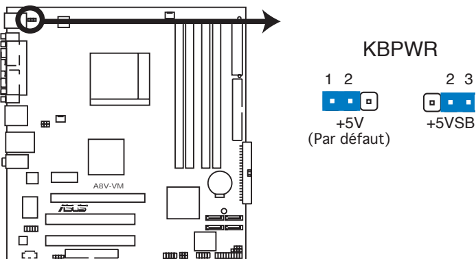
Paramètres d'alimentation du clavier de l'A8V-VM
