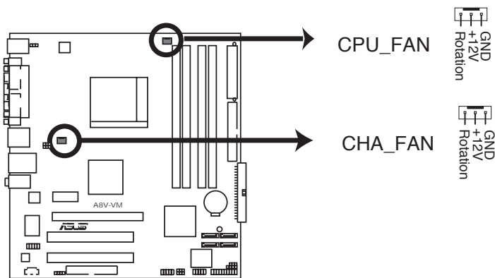
Connecteur ventilateurs de l'A8V-VM
