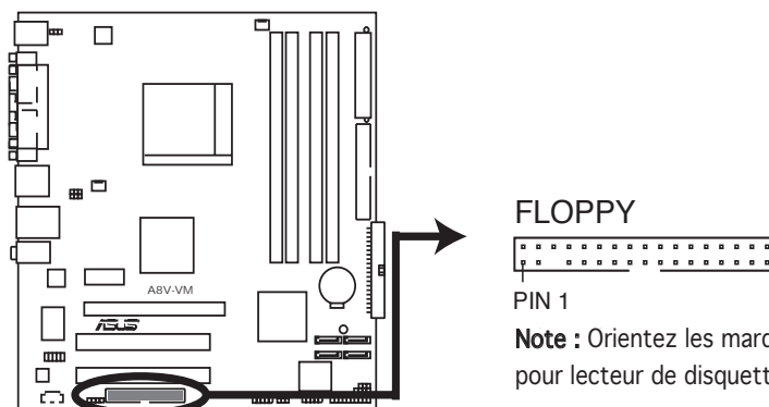
Connecteur lecteur de disquettes de l'A8V-VM
