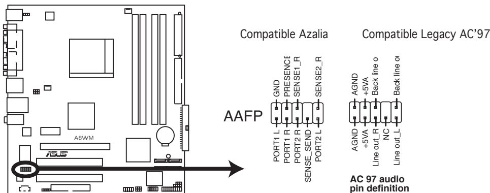
Connecteur Front panel audio de l'A8V-VM
