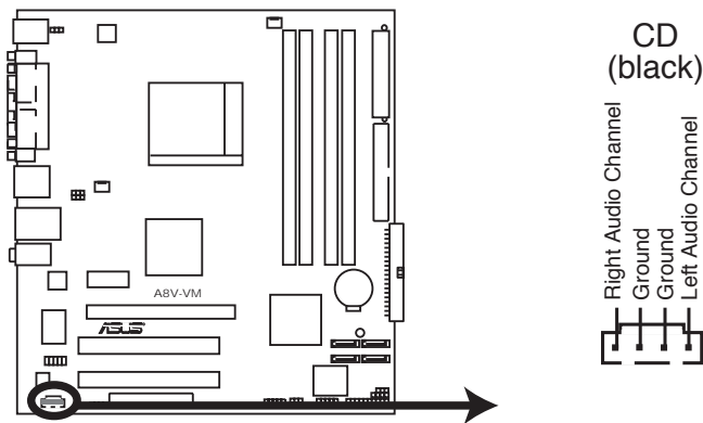
Connecteur audio interne de l'A8V-VM
