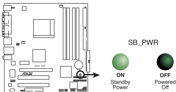
LED embarquée de l'A8V-VM
