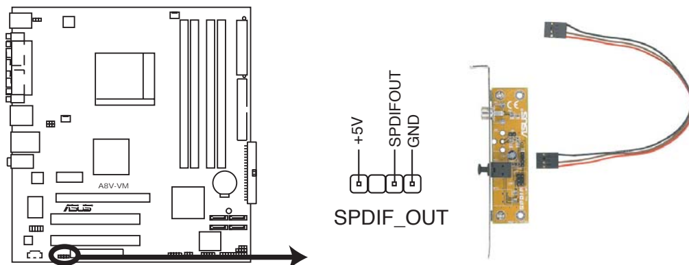
Connecteur audio numérique de l'A8V-VM
