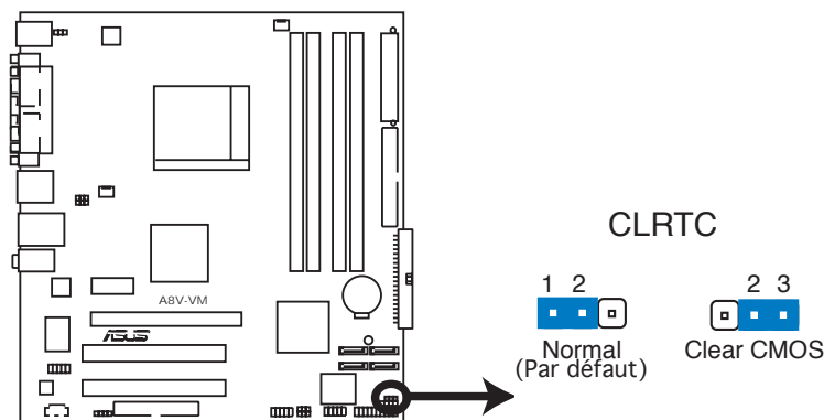
Clear RTC RAM de l'A8V-VM
