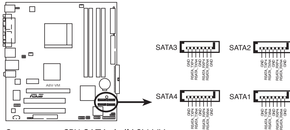
Connecteurs CPU SATA de l'A8V-VM
