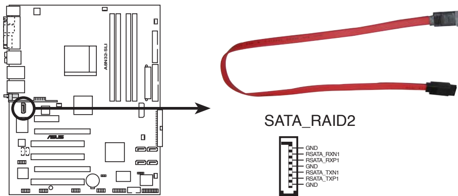
Connecteurs RAID SATA de l'A8N32-SLI DELUXE
