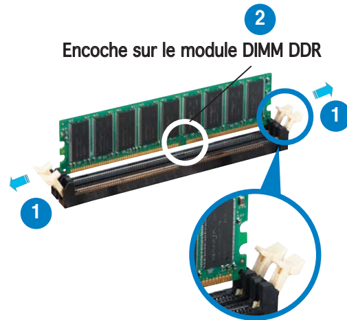
Clip de rétention déverrouillé
