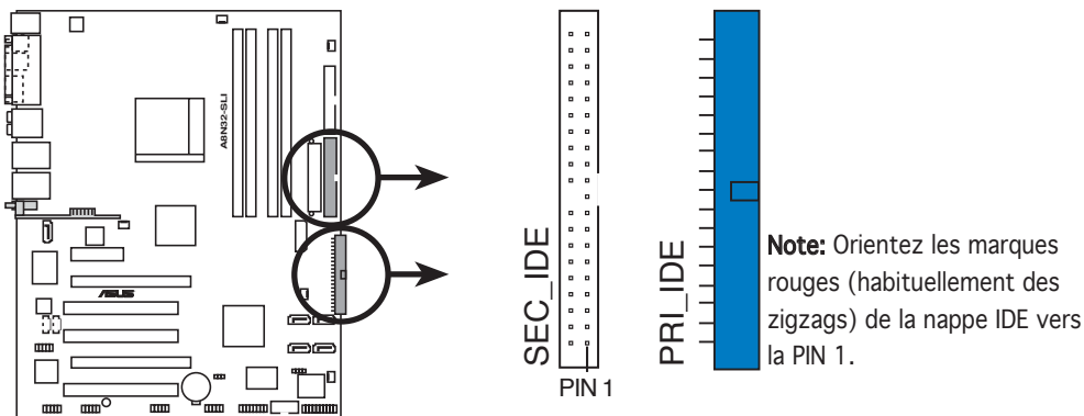
Connecteurs IDE de l'A8N32-SLI DELUXE
