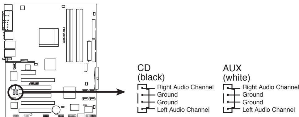
Connecteurs audio internes de l'A8N32-SLI DELUXE
