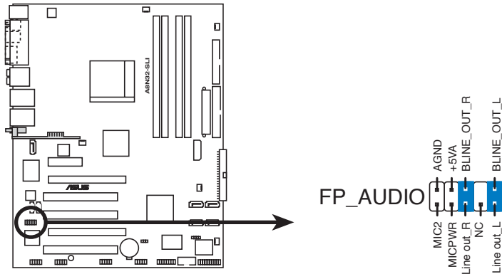
Connecteur Front panel audio de l'A8N32-SLI DELUXE
