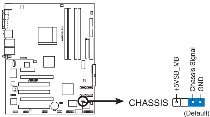
Connecteur Chassis intrusion de l'A8N32-SLI DELUXE
