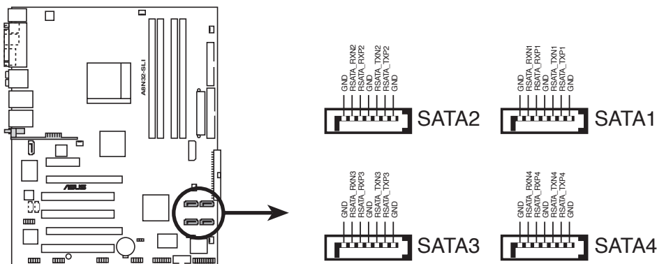
Connecteurs SATA de l'A8N32-SLI DELUXE
