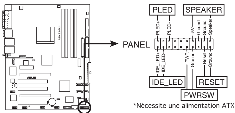
Connecteur System Panel de l'A8N32-SLI DELUXE
