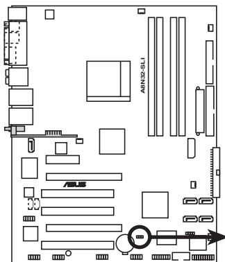
Clear RTC RAM de l'A8N32 SLI DELUXE
