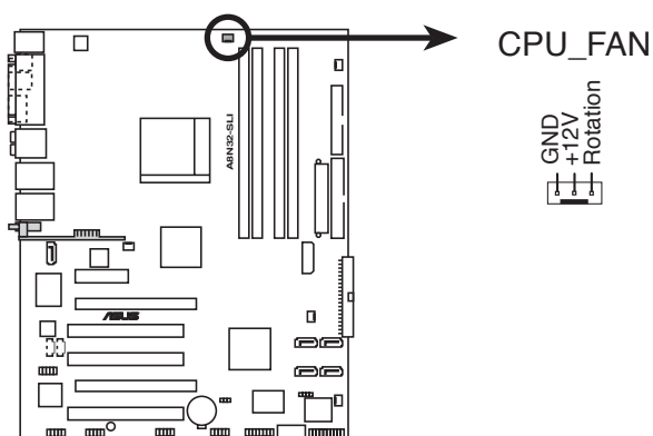
Connecteur du ventilateur CPU de l'A8N32-SLI DELUXE
