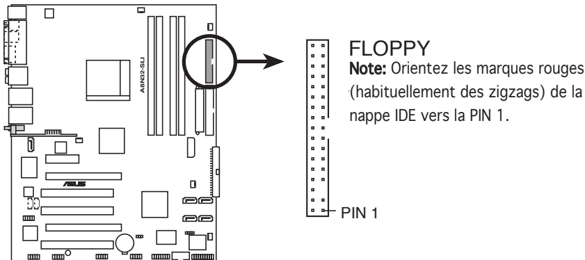
Connecteur lecteur de disquettes de l'A8N32-SLI DELUXE
