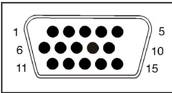
Connecteur signaux
