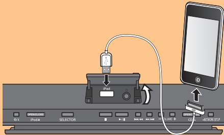
Câble dédié fourni avec le dispositif iOS
