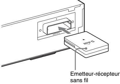
Panneau arrière de l'appareil
